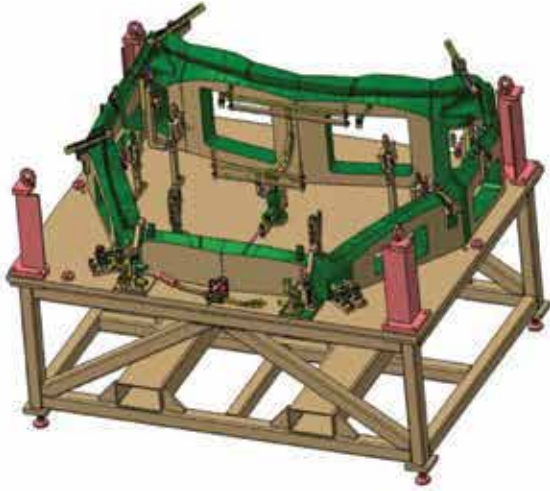
Frontklappe
