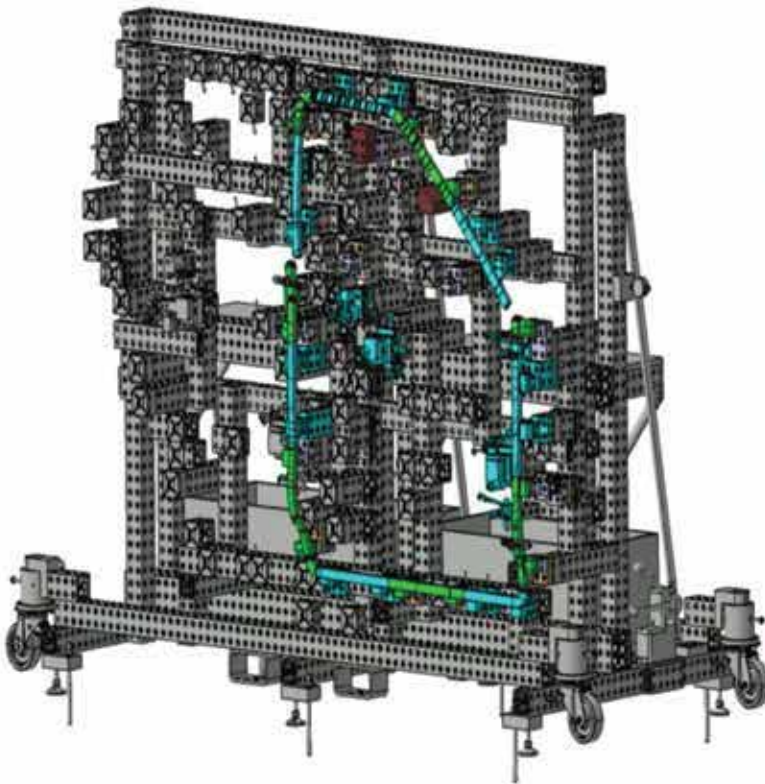
Tür Vorne
